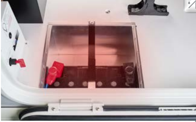
Batteriezentrale beheizt mit Batterie Hauptschalter; Serie: Gel-Batterien 1 x 80 Ah, erweiterbar auf 2 x 80 Ah, optional Lithium-Ionen-Batterie 90 Ah inklusive Batteriecomputer und separatem Touch-Display
